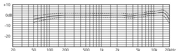
Frequenzgang mit Toleranzfeld
