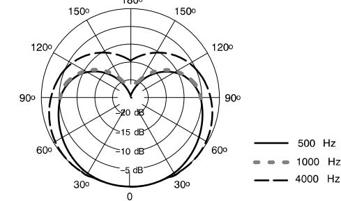
TYPISCHE RICHTCHARAKTERISTIK ABBILDUNG 3
