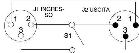
SCHEMA CIRCUITALE DELL'INTERRUPTORE DI ALIMENTAZIONE FIGURA 6
