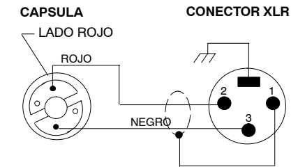
DIAGRAMA DE ALAMBRADO DEL SM10A FIGURA 4
